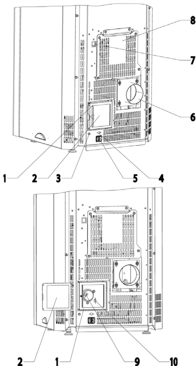
Abbildung 1: Anschlüsse hinten
