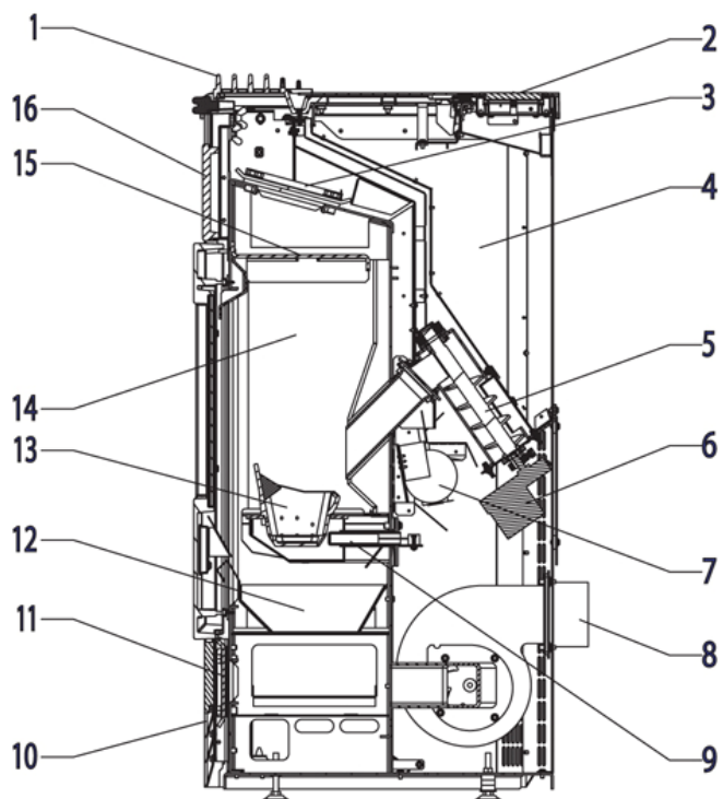
Abbildung 29:: Ersatzteile 302.06 / 309.06
