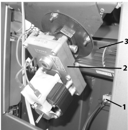
Abbildung 11: Schneckenmotor
