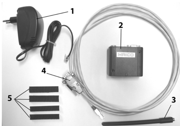
Abbildung 21: Teileliste GSM Modul
