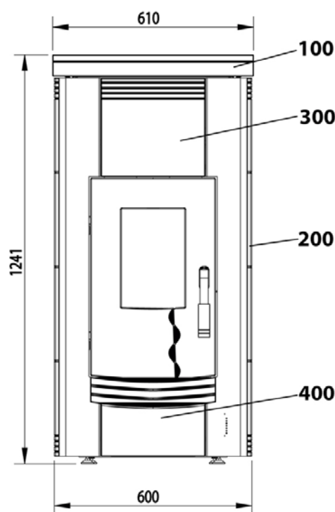
Abbildung 30: Ersatzteile und Abmessungen 302.07C
