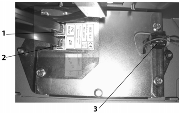
Abbildung 15: Bedieneinheit Unterseite
