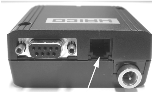
Abbildung 26: Anschluss Steckernetzteil
