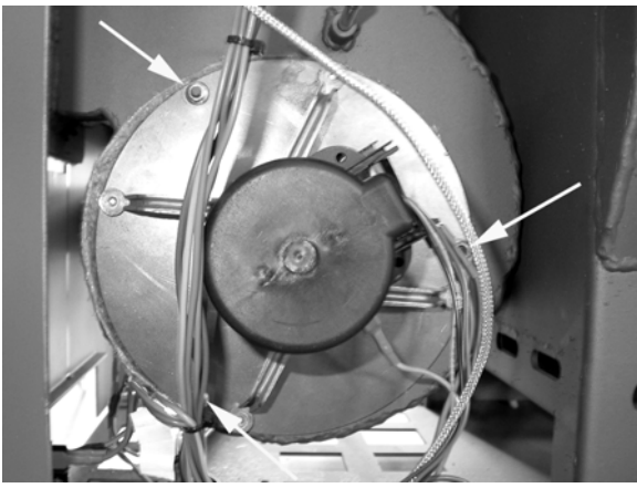
Abbildung 10: Abgasventilator
