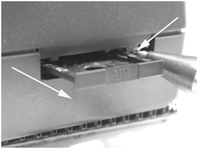
Abbildung 25: Einlegen SIM-Karte
