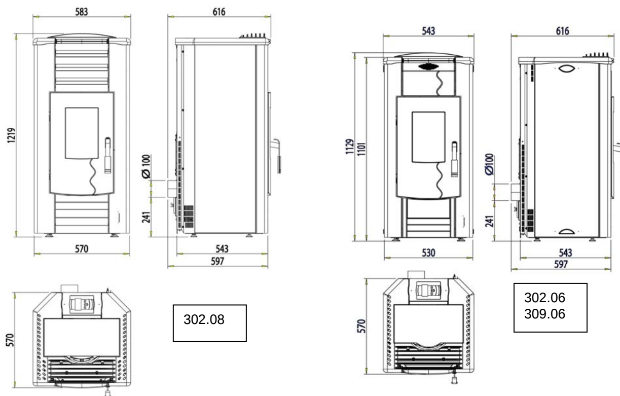
Abbildung 27: Abmessungen
