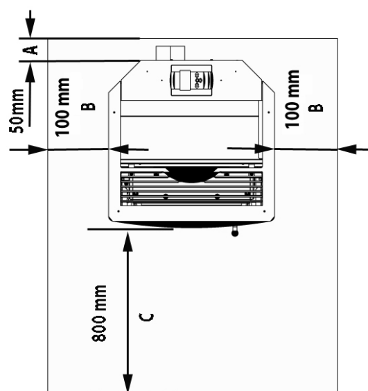
Abbildung 2: Sicherheitsabstände
