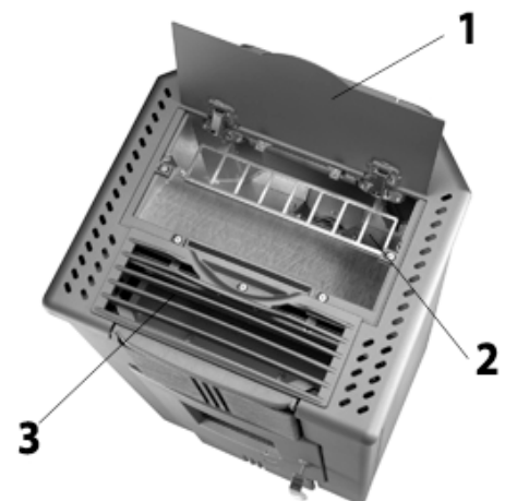
Abbildung 7: Pellettank
