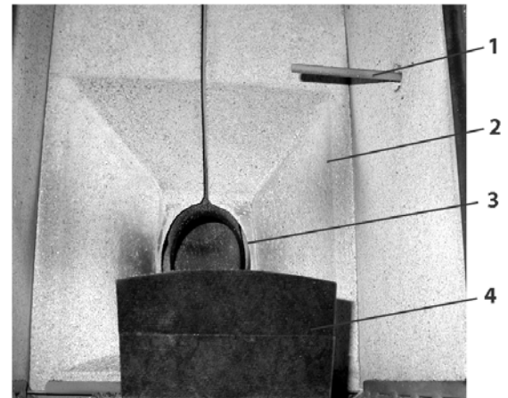
Abbildung 18 : Brennraum
