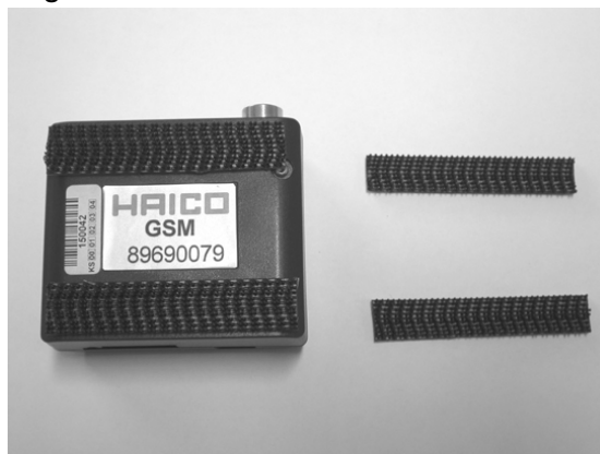
Abbildung 24: Montage GSM Modul
