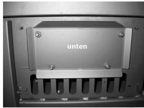
Abbildung 8c: Reinigungsdeckel unten
